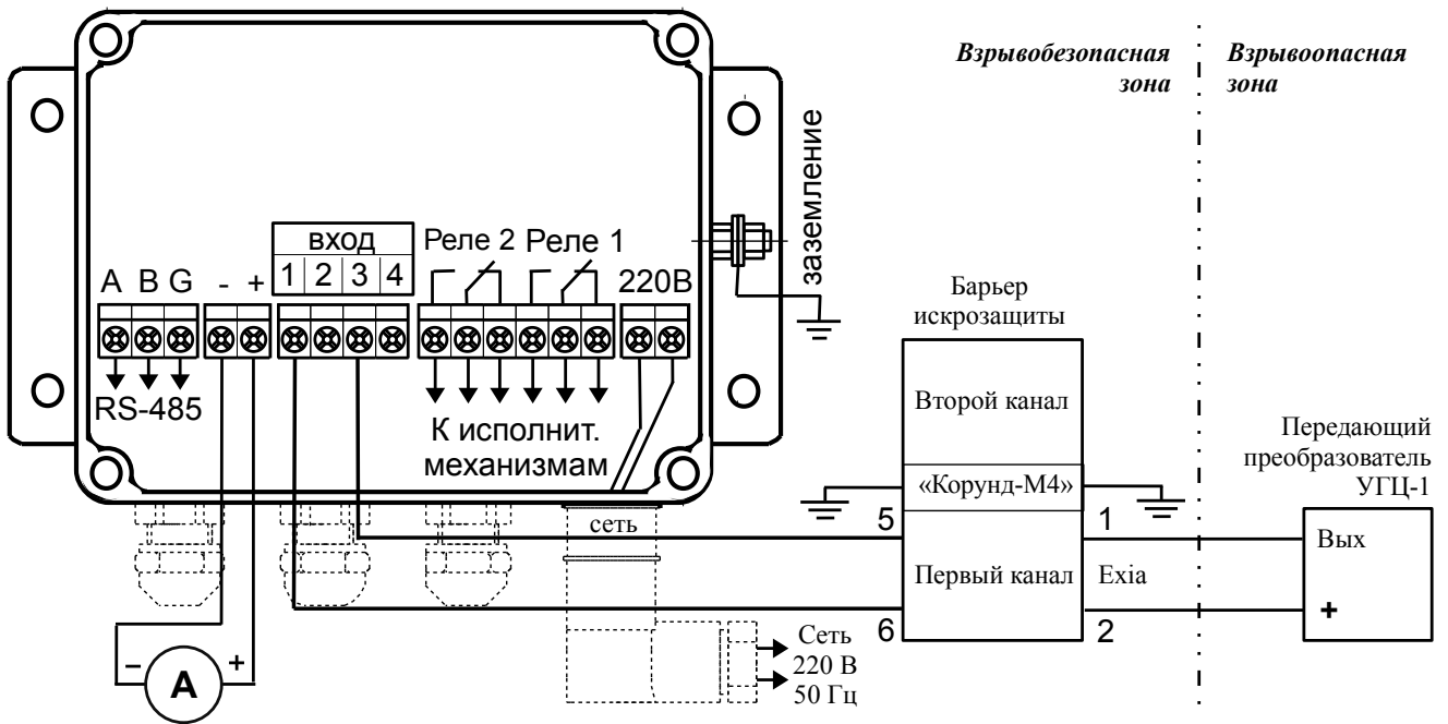
б) УГЦ-1.х-Ех с измерительным прибором настенного исполнения (крышка снята)
