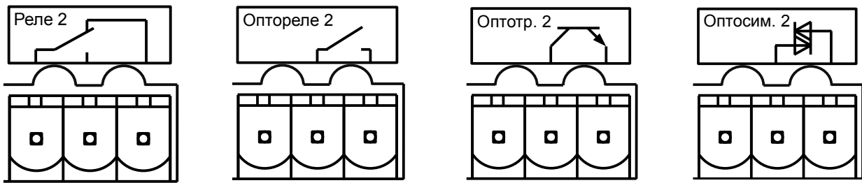
а) электромагнитное реле (сухой контакт)
