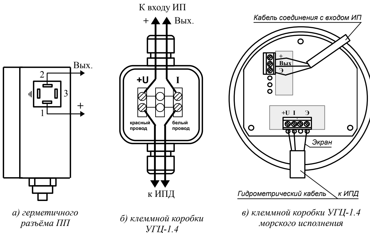
Рисунок Г.1 - Назначение контактов
