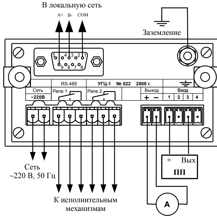
а) для исполнения без БВД-8
