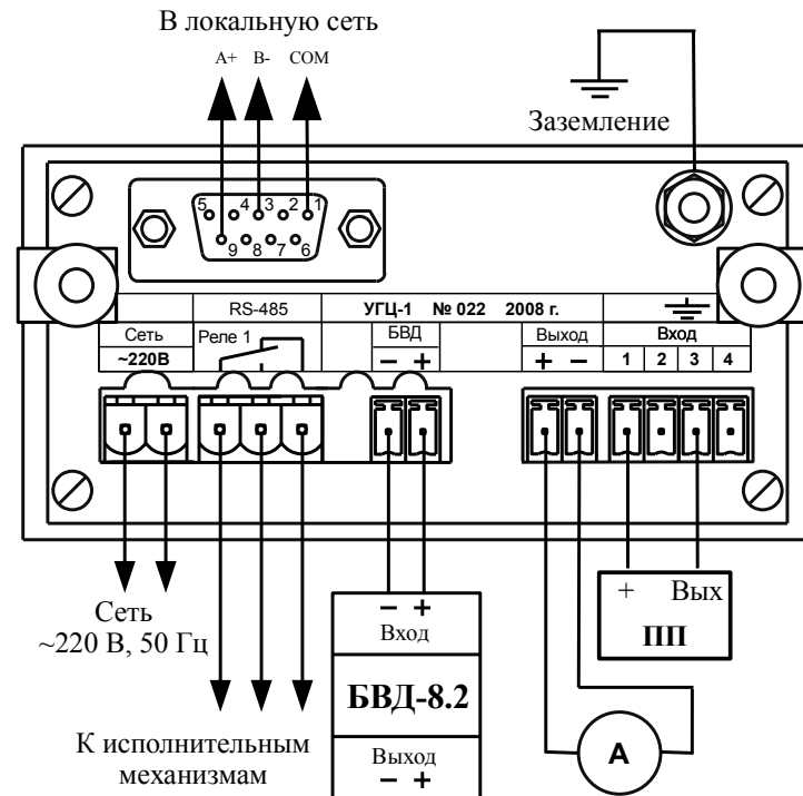
б) для исполнения с БВД-8
