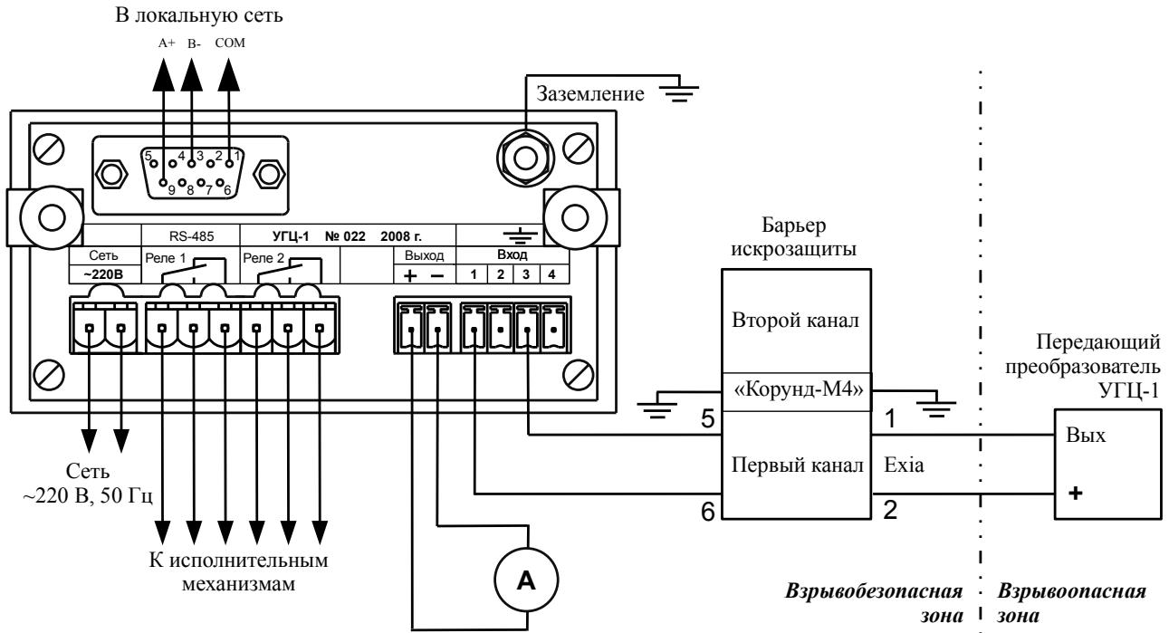
а) УГЦ-1.х-Ех с измерительным прибором щитового исполнения
