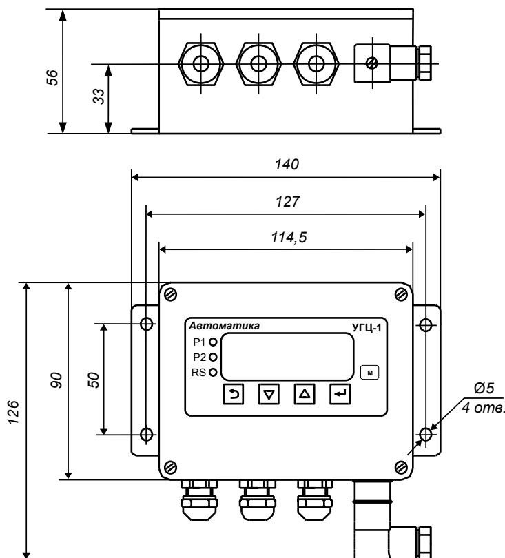
Рисунок А.2 - Измерительный прибор настенного исполнения
