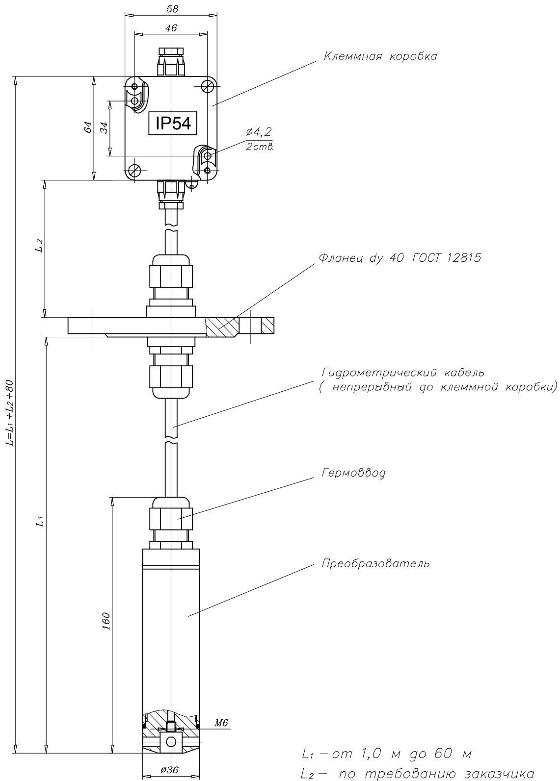
Рисунок Б.4 - Передающий преобразователь УГЦ-1.4, УГЦ-1.4-Ex
