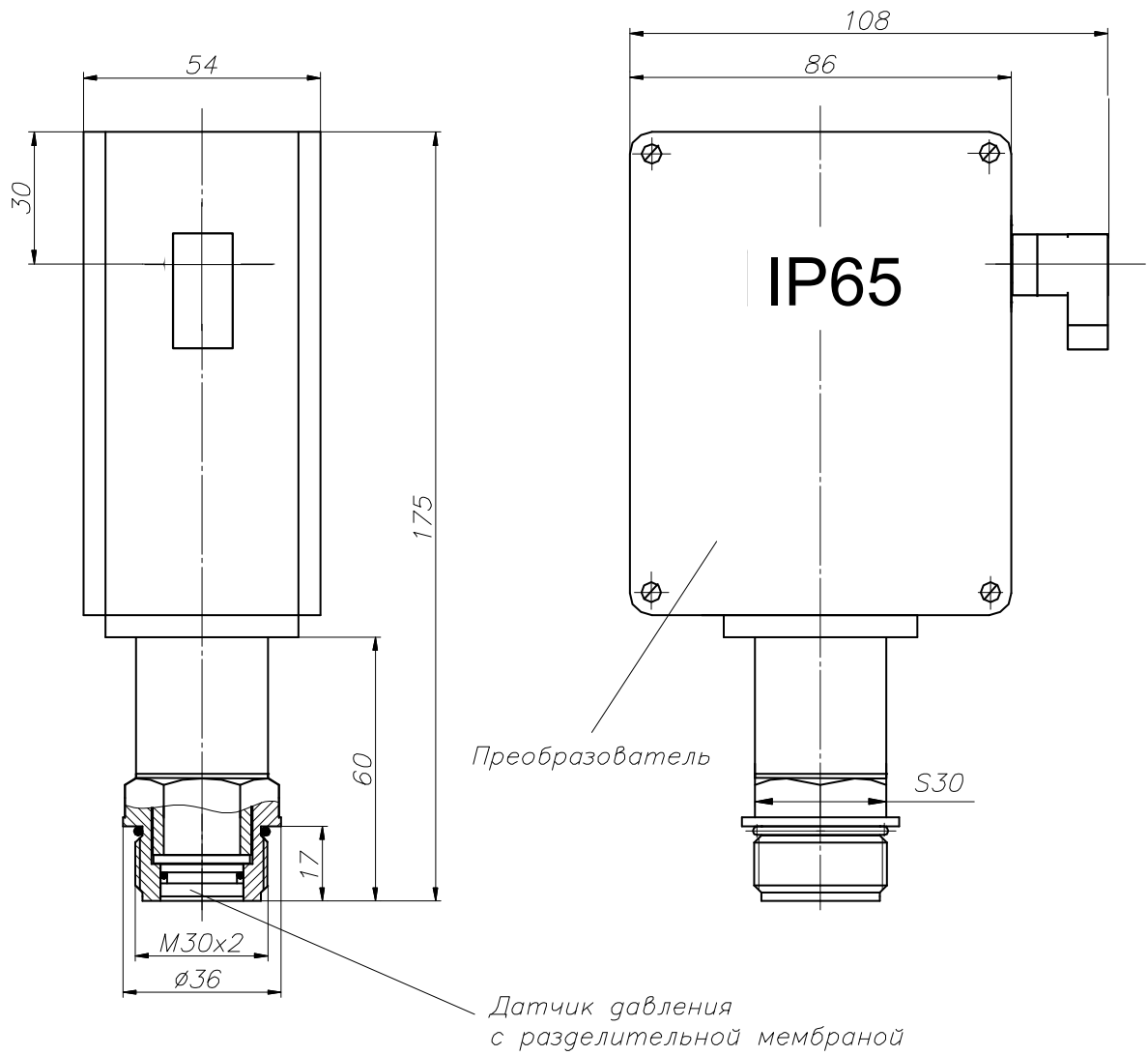
Рисунок Б.3 - Передающий преобразователь УГЦ-1.3, УГЦ-1.3-Ex
