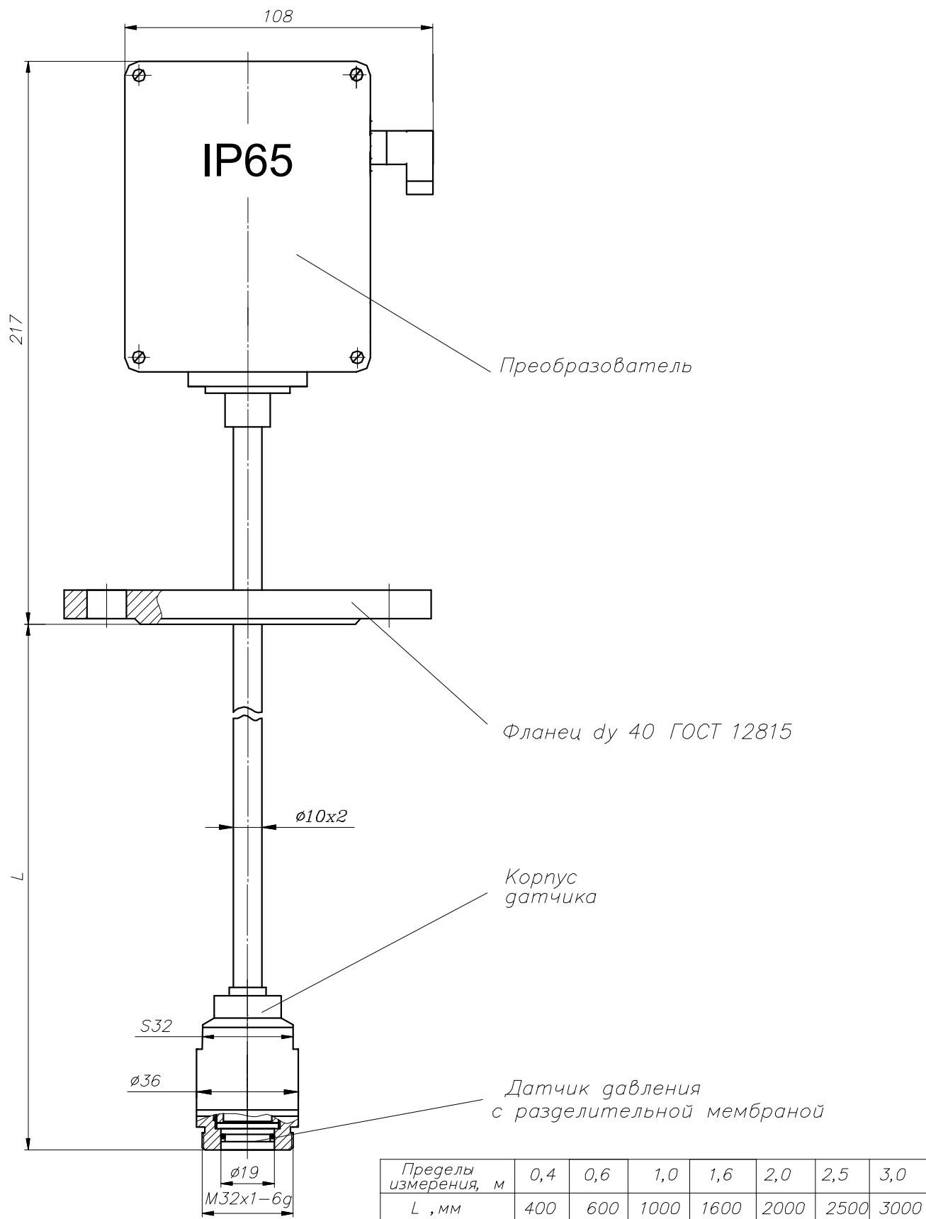
Рисунок Б.6 - Передающий преобразователь УГЦ-1.5, УГЦ-1.5-Ех
